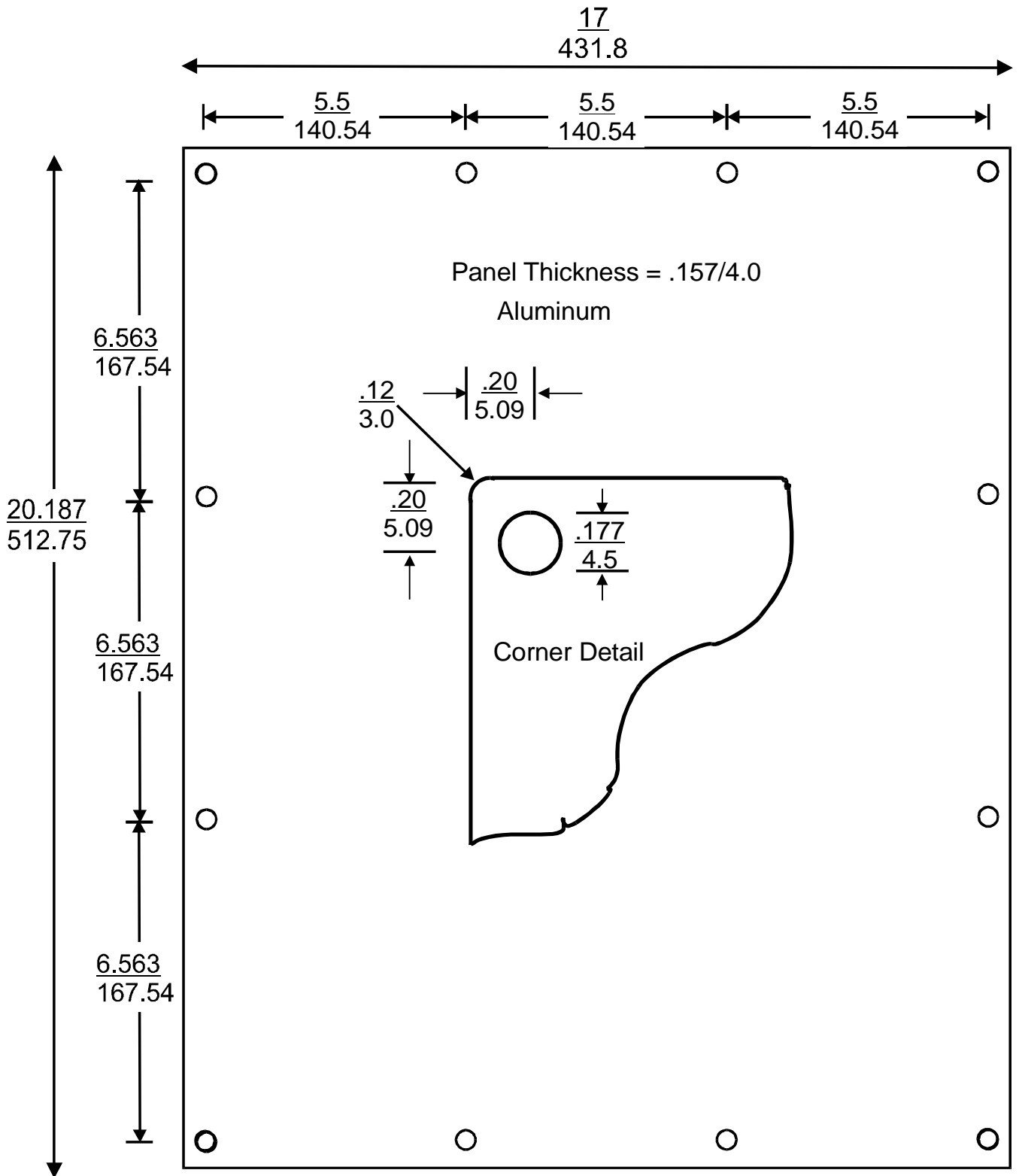
M267 Dimensions
